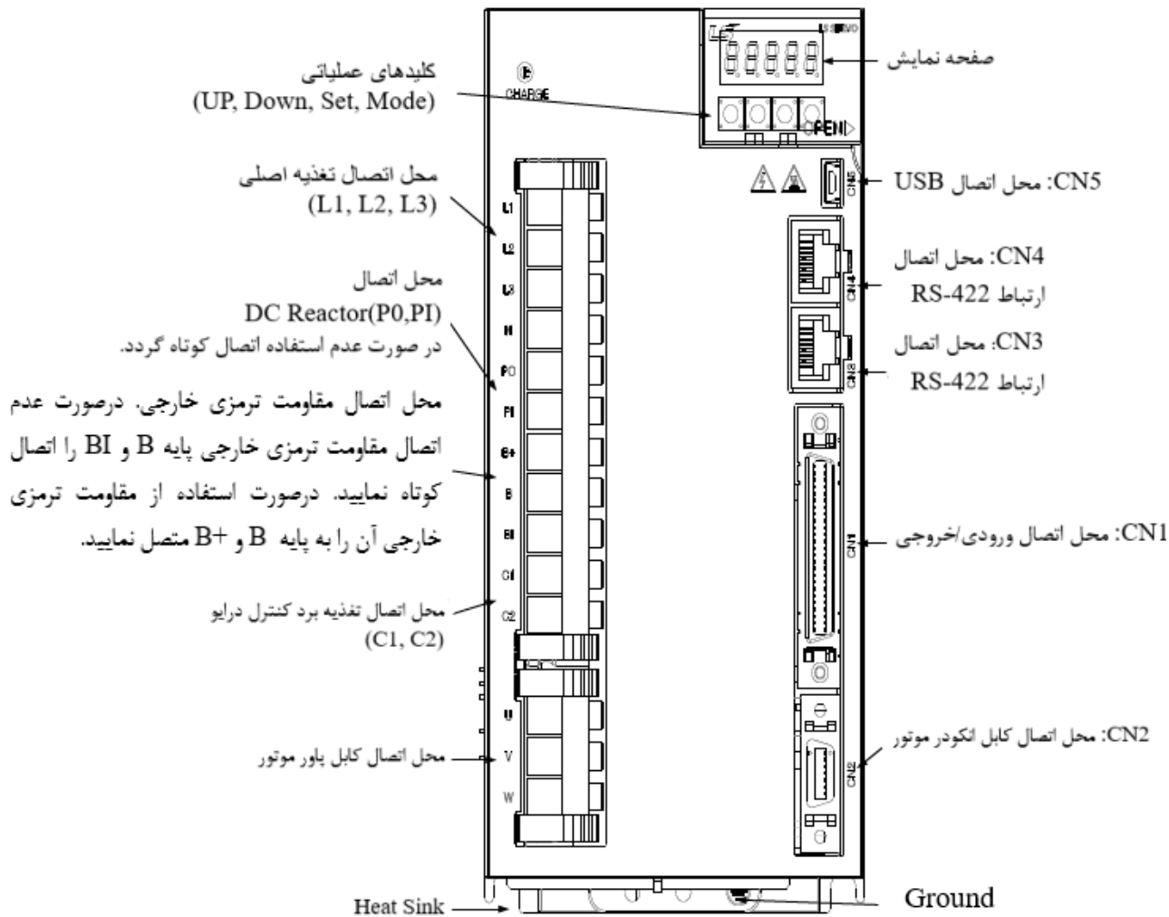
سروو درایو L7SA020, L7SA035
