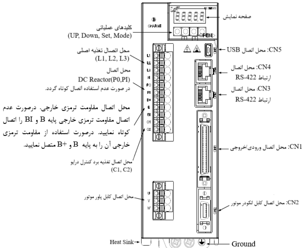
سروو درایو L7SA008, L7SA010
