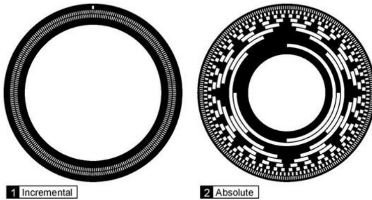
انکدر مطلق (Absolute) و افزایشی (Incremental)
