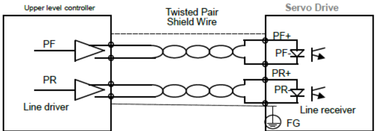
-1 بصورت Line drive با ولتاژ 5 ولت
