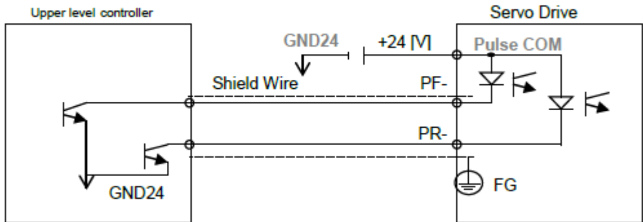
-2 بصورت open collector NPN 24(V)
